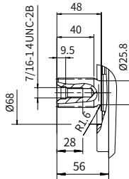
“B4” 型花键轴 ANSI B92.1b 1 1/4 in 14T 12/24DP
