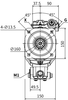
X向视图
