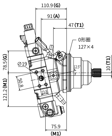
X向视图
