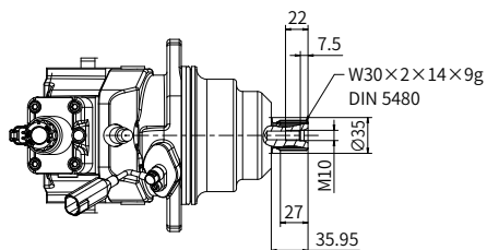
Y向视图
