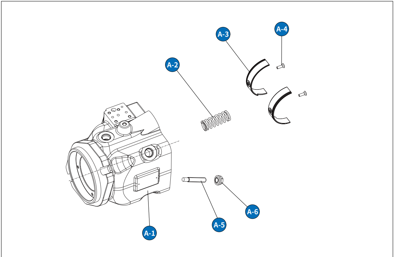
壳体部件清单
